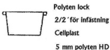
Rektangulär ponton
